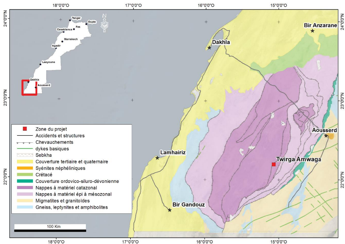
Localisation et contexte géologique général de Twirga-Amwaga
