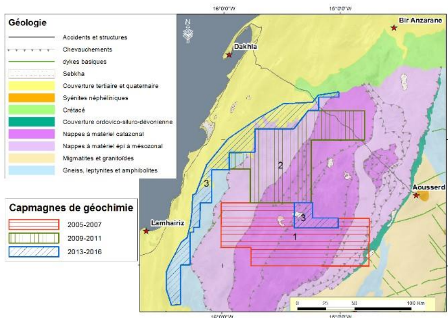
Carte de situation et cadre géologique général de la zone d'étude
